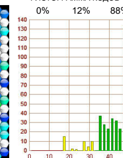
ГИСТОГРАММА КОДОВ
