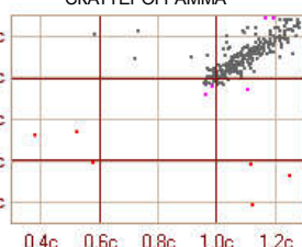
СКАТТЕРОГРАММА
